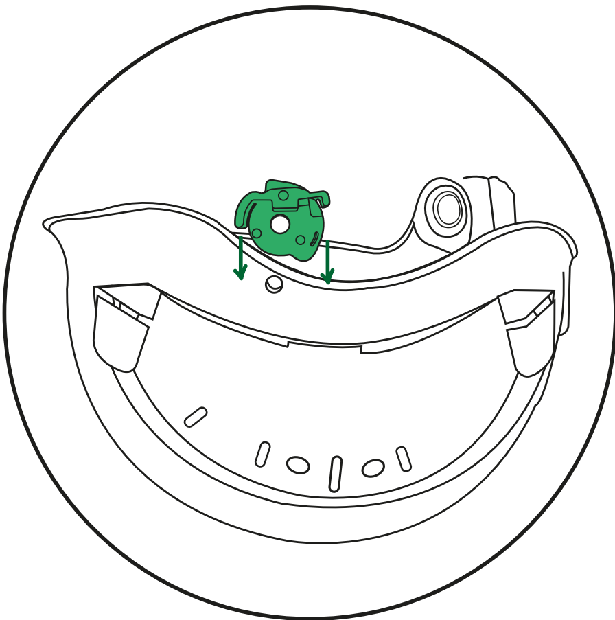
2 AJUSTAR PIEZA 2
