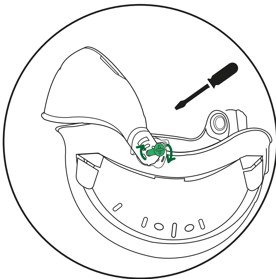
4 INTRODUCIR TORNILLO
